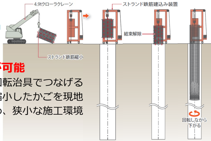
施工ステップ（工場組立縮小、現場伸展方式）
